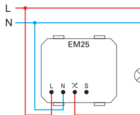
(2) három vezetékű csatlakozás three-wire connection
