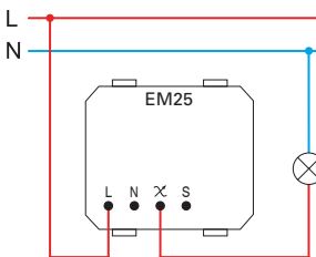
(1) két vezetékű csatlakozás two-wire connection
